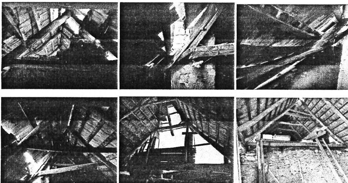
Tetőszerkezet részletei
